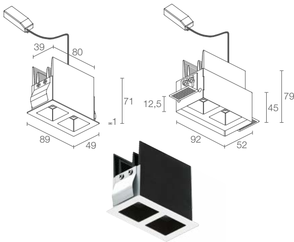
Cassaforma per installazione arretrata non inclusa
