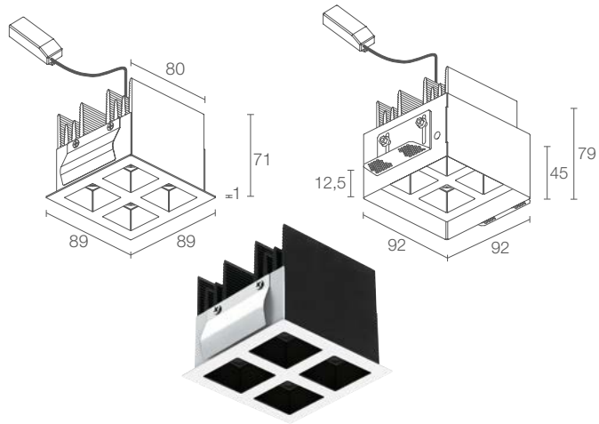
Cassaforma per installazione arretrata non inclusa
