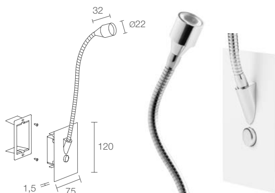
Stelo flessibile: Ø8 mm - 400 mm
